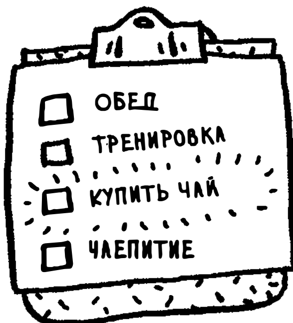
Упорядоченный
