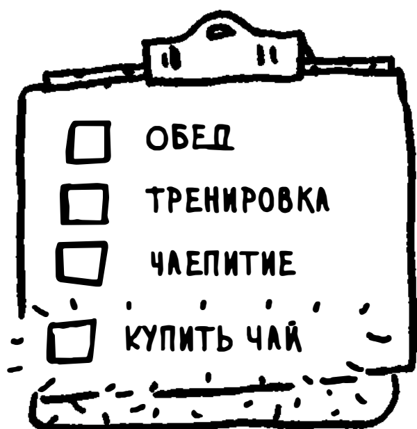
Неупорядоченный
