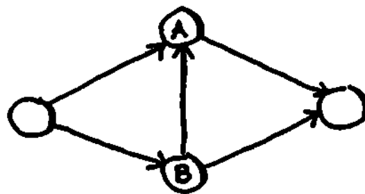
НЕВЗВЕШЕННЫЙ ГРАФ
