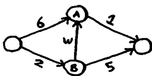
ВЗВЕШЕННЫЙ ГРАФ
